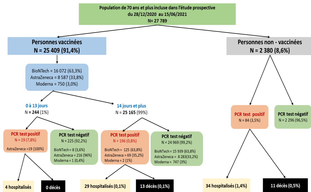
Figure 1 Flow chart des données du 28/12/2020 au 15/06/2021
