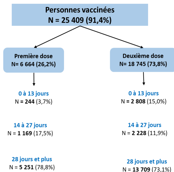
Figure 2 Flow chart des personnes vaccinées selon leur statut vaccinal et intervalles post-vaccination
